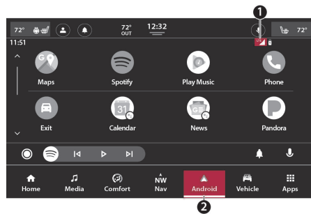
Android Auto™
